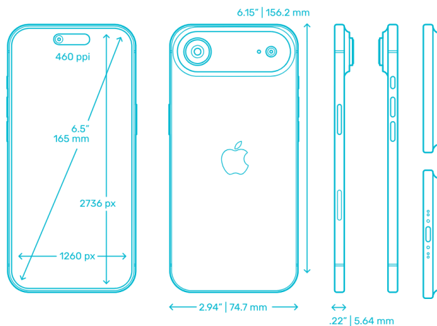
Figura 1. Dimensiones físicas del iPhone Air.
